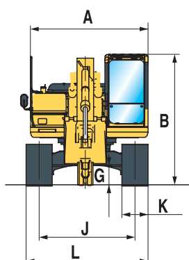
MONOBLOCK-AUSLEGER
