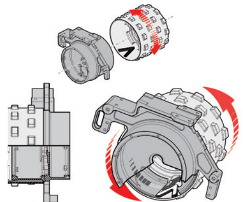
Integrierte Bandagenabstreifer
