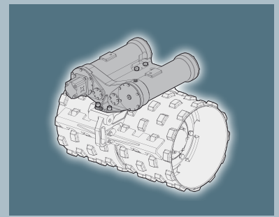
Leicht zugängliche Unwuchteinheit mit SCT (Straight Compaction Technology)
